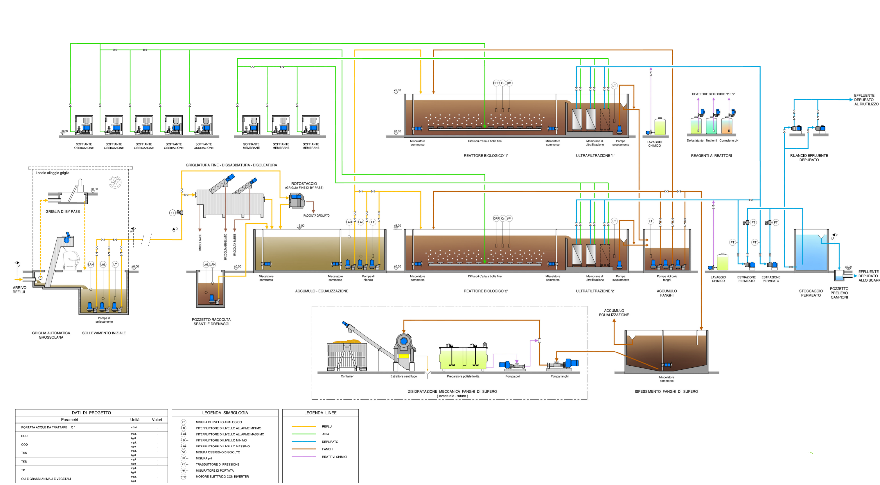
SCHEMA TECNOLOGICO FUNZIONALE DELL'IMPIANTO DI DEPURAZIONE
