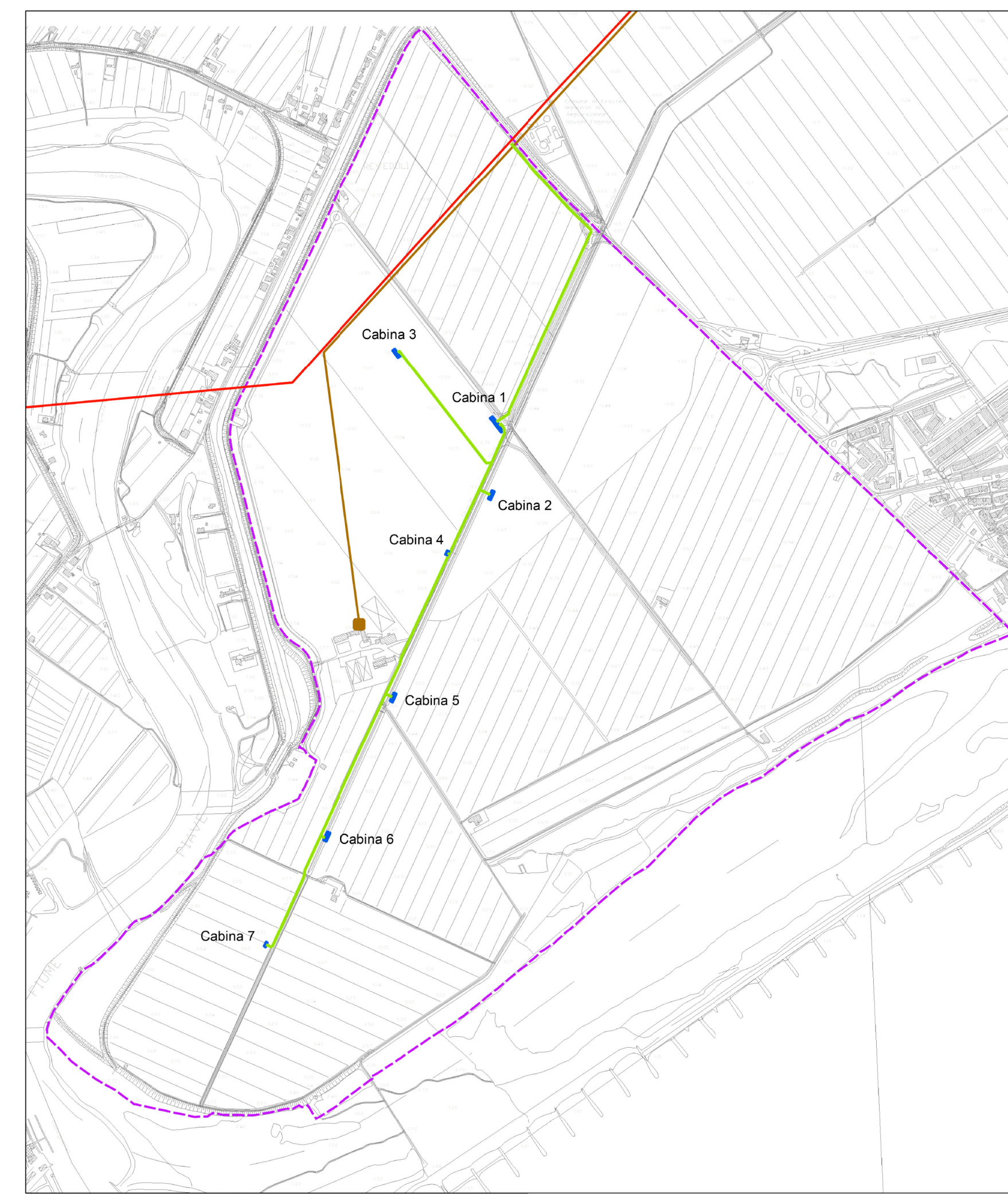
SCHEMA DELLA DISTRIBUZIONE RETE MT - scala 1:10000
