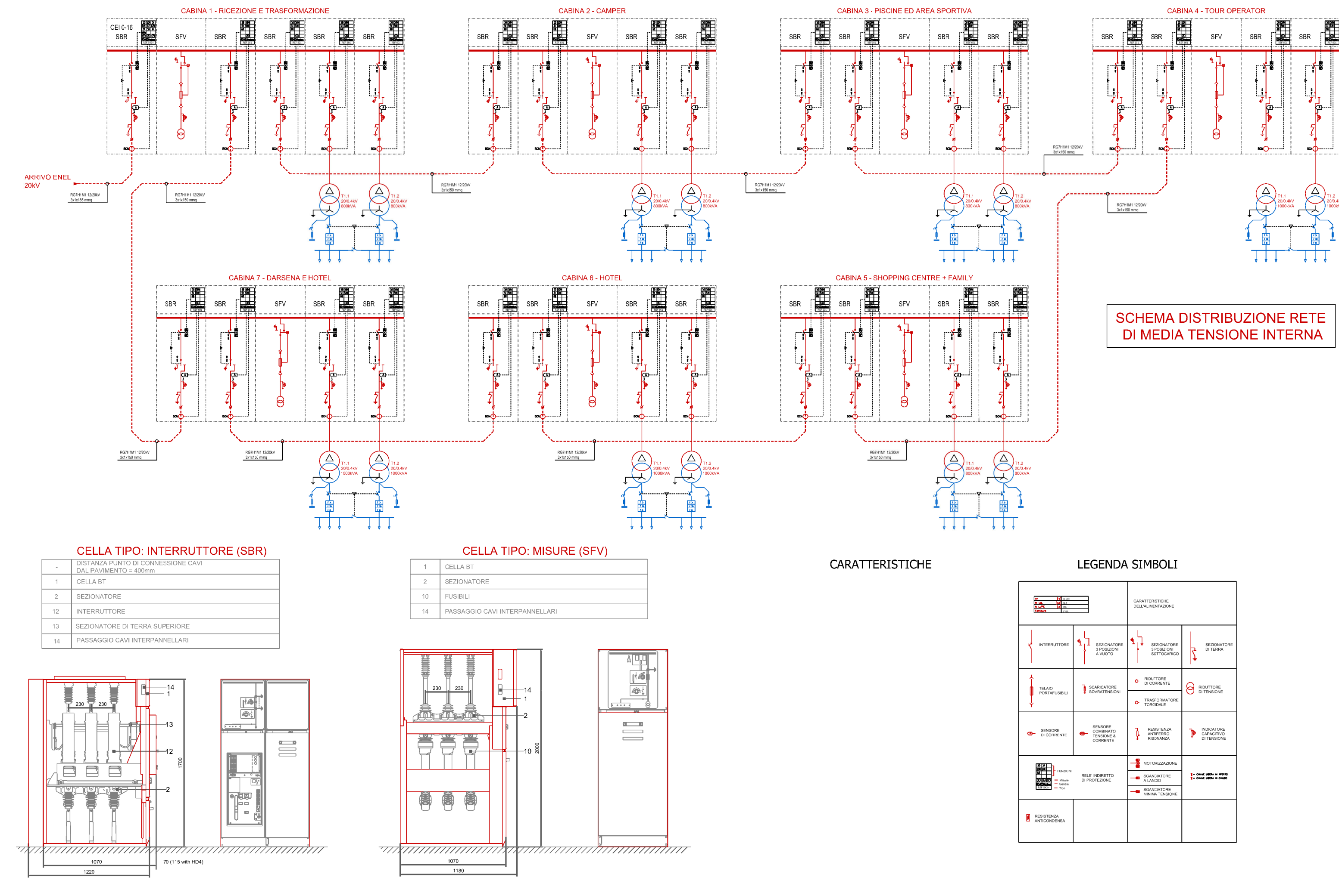
SCHEMA UNIFILARE RETE MT
