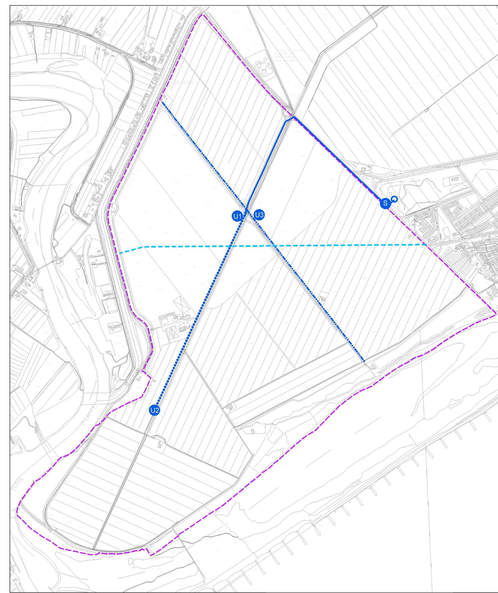
SCHEMA DELLA RETE ACQUEDOTTISTICA - scala 1:10000
