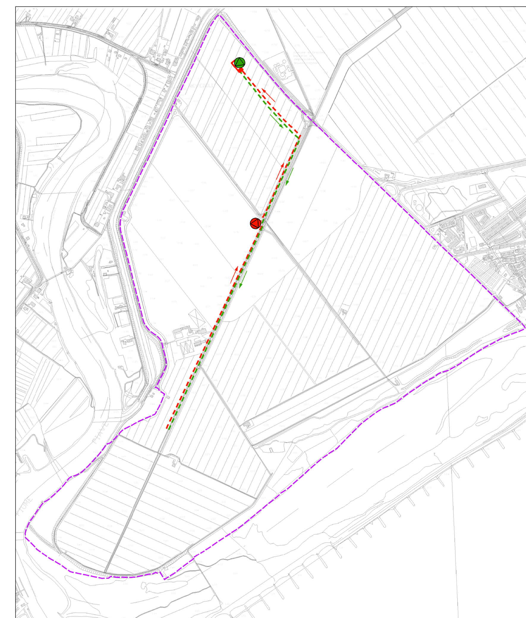
SCHEMA DELLA RETE DI SCOLO DELLE ACQUE METEORICHE - scala 1:10000
