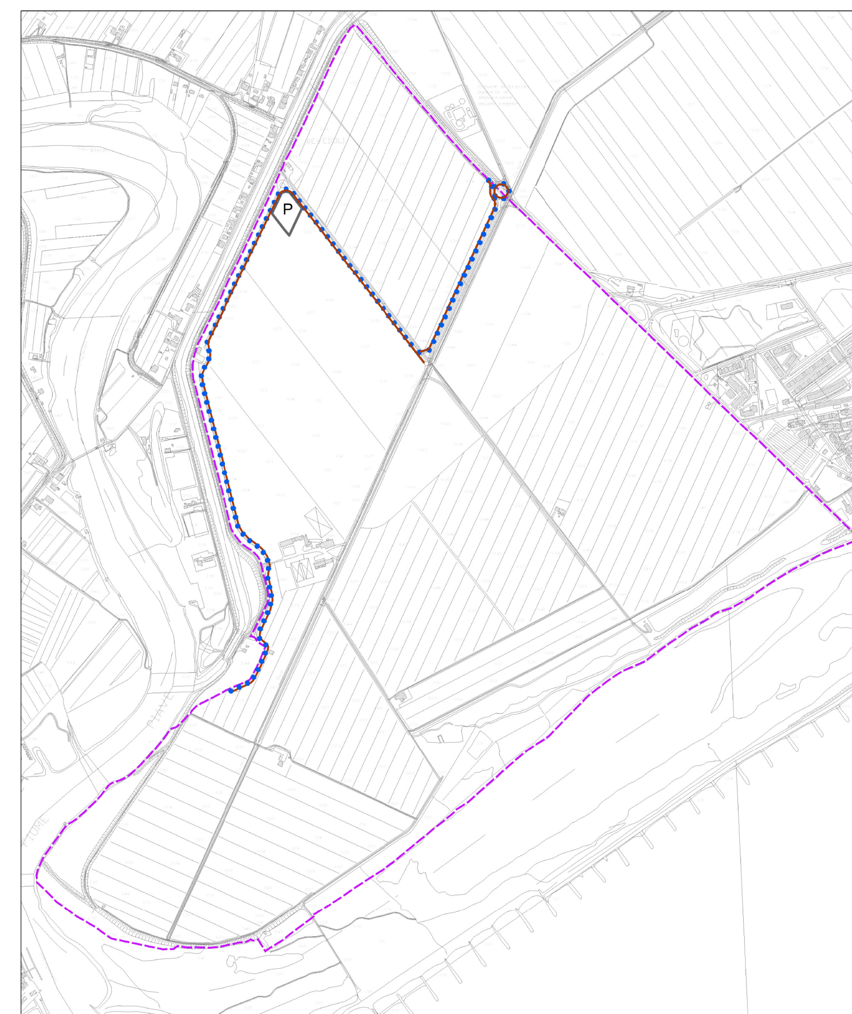
SCHEMA DELLA RETE DELL'ILLUMINAZIONE PUBBLICA - scala 1:10000
