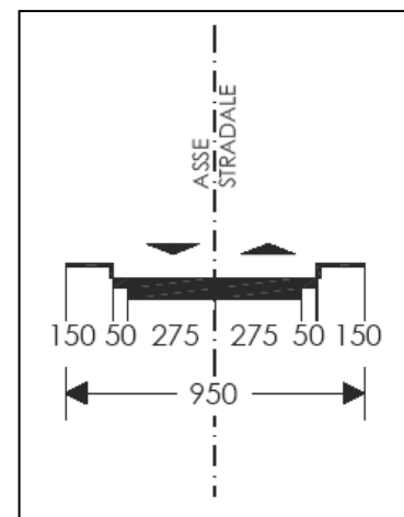
Sezione base a 2) 1 corsia per senso di marcia
