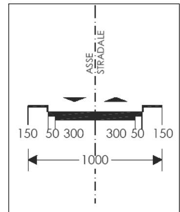
Sezione base a 1) 1 corsia per senso di marcia
